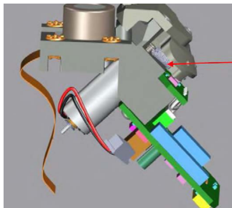
Ressort de rappel
