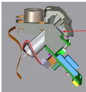
Ressort de l'obturateur
